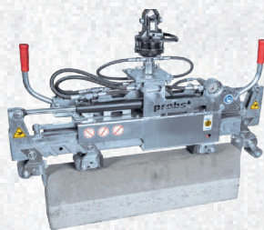
POSE BORDURE HYDRAULIQUE pour pelles 2.5T à 3T
